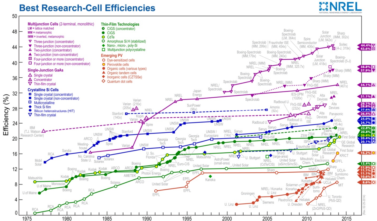
شکل ۱۱- بازده سلول‌های خورشیدی به‌عنوان تابعی از زمان با استفاده از تکنولوژی‌های مختلف فوتولتائی در طول فرآیند پیشرفت (منبع: آزمایشگاه ملی انرژی‌های تجدیدپذیر ایالات متحده)
