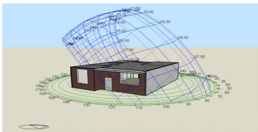
شکل ۱- مدل هندسی ساختمان مسکونی مورد مطالعه در نرم‌افزار دیزاین‌بیلدر.
