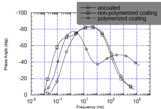
شکل ۷- نمودار بد-فاز تست امپدانس الکتروشیمیایی آلومینیم پوشش داده شده و بدون پوشش [۱۳].
