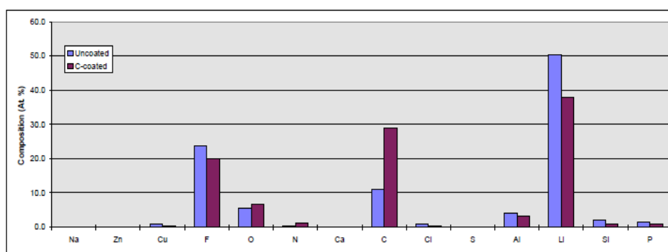
شکل ۹- مقایسه نتایج تست آنالیز XPS بر روی آلومینیم پوشش داده شده بعد از ۲۱۲ سیکل شارژ و دشارژ در الکترولیت باتری [۱۴].
