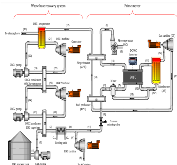
شکل ۳ - شماتیک سیستم ارائه شده با یک ترکیب ORC حلقه دوگانه برای بازیابی گرمای زباله از SOFC مجهز به توربین گازی
