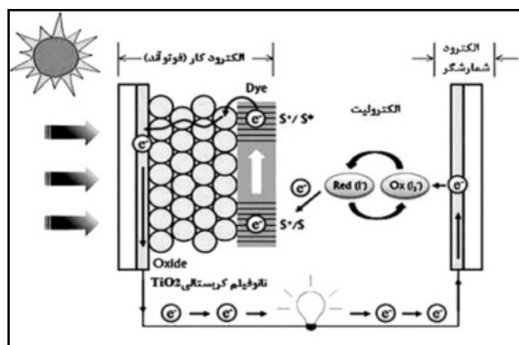
شکل ۸- طرح شماتیکی از عملکرد سلول حساس شده به رنگ‌دانه [۲۱]
