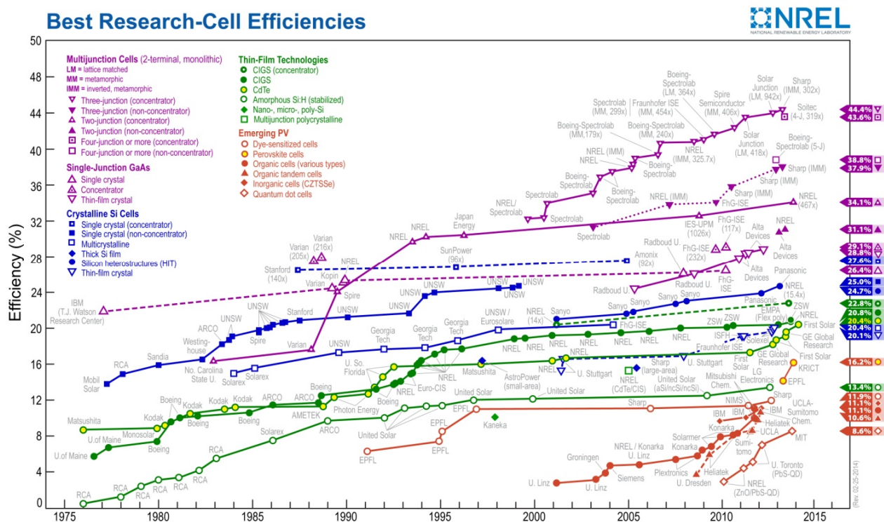
شکل ۱۱- بازده سلول‌های خورشیدی به‌عنوان تابعی از زمان با استفاده از تکنولوژی‌های مختلف فتوولتائی در طول فرآیند پیشرفت (منبع: آزمایشگاه ملی انرژی‌های تجدیدپذیر ایالات متحده)
