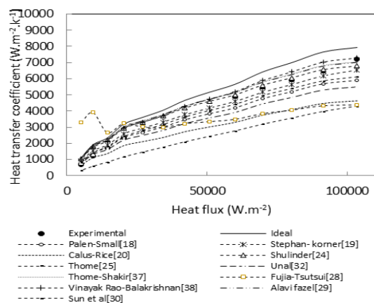
نمودار ۵: مقایسه‌ی نتایج آزمایشگاهی ضریب انتقال حرارت غلظت مولی ۰/۰۸ محلول آب و اتانول با روابط موجود
