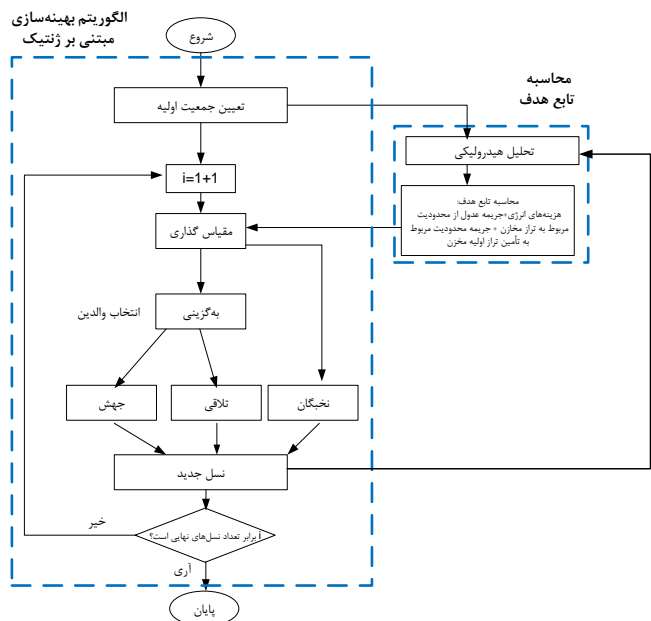
شکل ۱- فلوچارت مدل کامپیوتری تعیین دستوالعمل نحوه بهره‌برداری بهینه از ایستگاه‌ها
