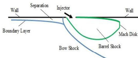
شکل ۲۷. تصویر شماتیک فیزیک تزریق جریان درون تونل
