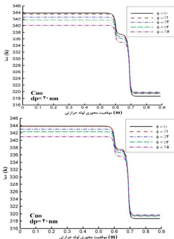
شکل ۷. اثر کسر حجمی و قطر ذرات بر توزیع دمای سطح دیواره لوله حرارتی برای قطرهای متفاوت
