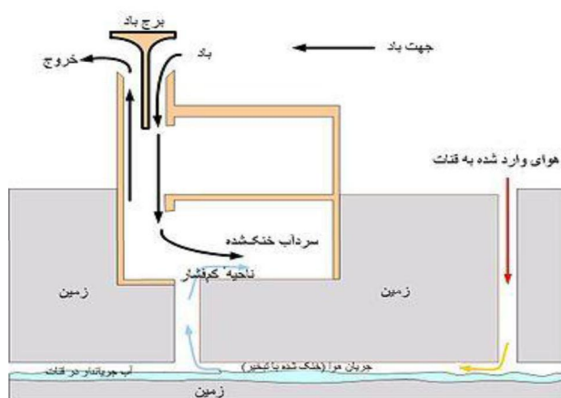
شکل ۱. مکانیزم سازه های بادگیر
