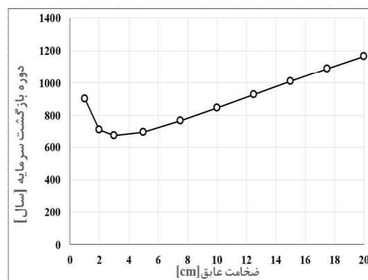
شکل ۹- تغییرات دوره بازگشت ساده سرمایه برحسب ضخامت عایق دیوارهای خارجی.
