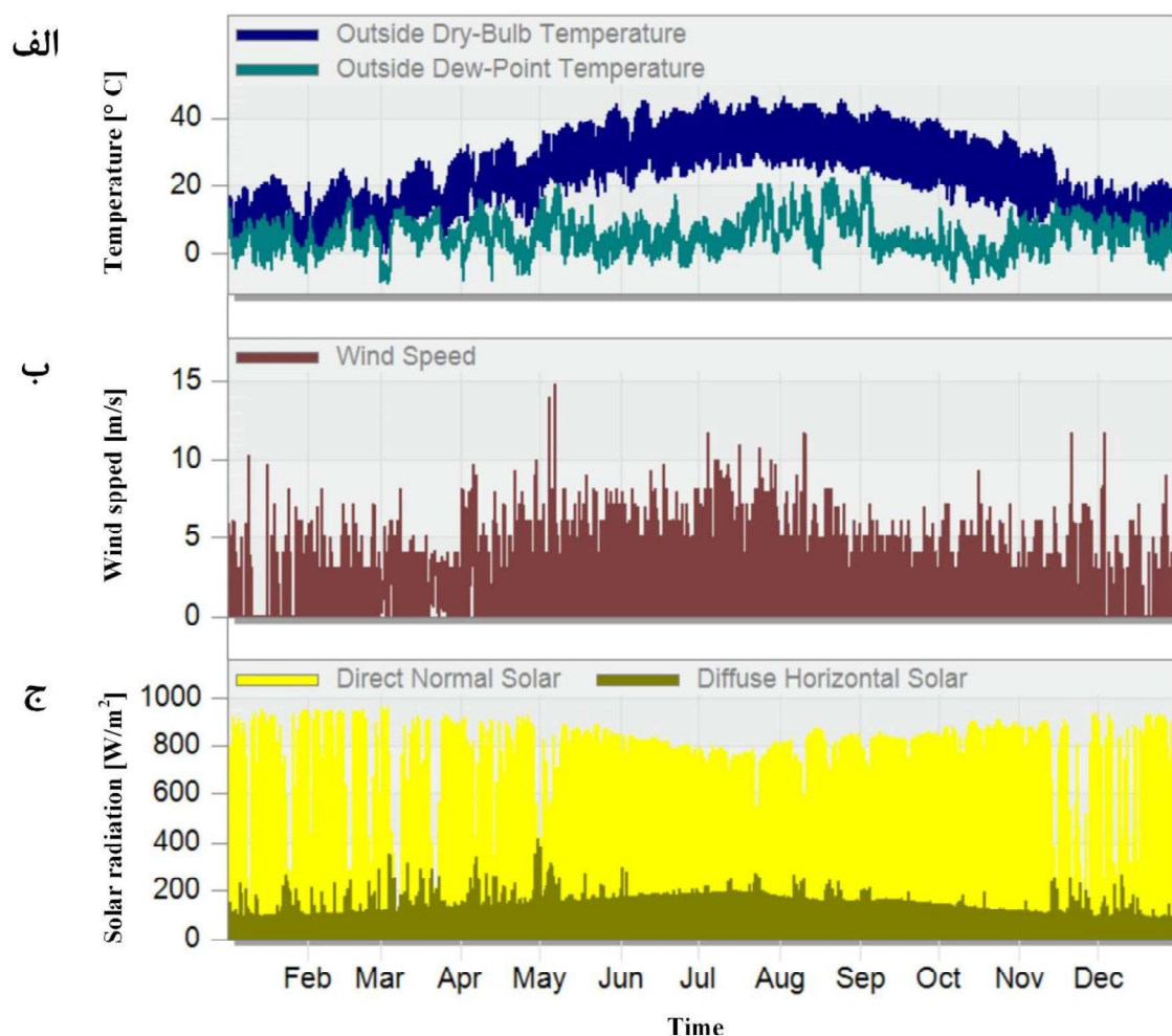
شکل ۲- تغییرات ساعتی پارامترهای اقلیمی شهر گچساران در طول سال الف) دمای خشک و دمای نقطه شبنم هوا ب) سرعت باد ج) تابش مستقیم و پخشیده خورشیدی.
