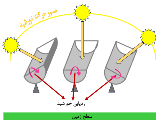
شکل ۶- تغییر محل قرارگیری خورشید در زمان‌های مختلف.
