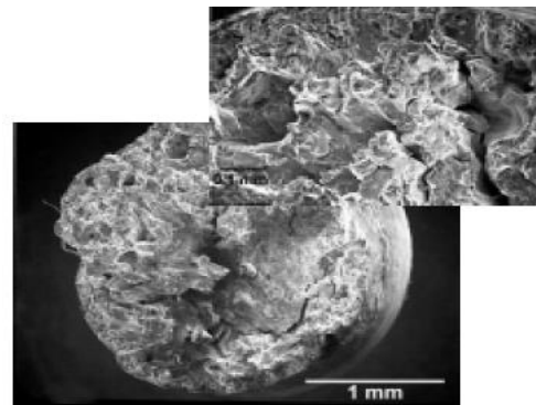
شکل ۱۴- تصاویر میکروسکوپ الکترونی از سطح ترک ایجاد شده در مس با دانه‌های درشت و کار سرد شده [۱۸].
