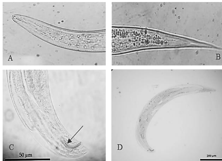
شکل ۱. نمای میکروسکوپی از سر (A) و دم (B) لارو سن دوم و نر بالغ (C) و اسپیکول نر (D) در گونه منتخب Steinernema carpocapsae .
