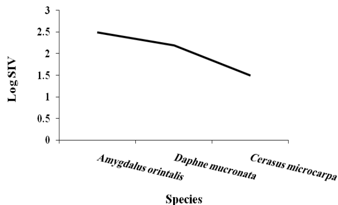
شکل ۱- مقادیر SIV گونه‌های درختچه‌ای در جهت شمال شرقی
