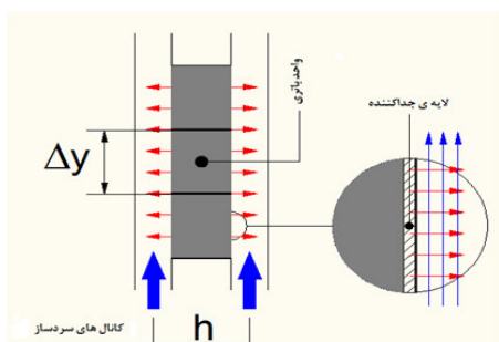
شکل ۲- نمایی از یک واحد باتری به همراه کانال‌های سرساز و لایه‌ی جداکننده‌ی مربوطه
