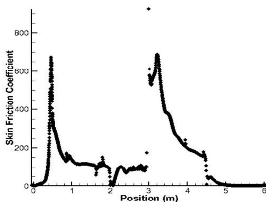
شکل ۲۰. نمودار ضریب اصطکاک در راستای محور تونل باد مجهز به انرژی
