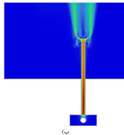
شکل ۶- مقایسه کانتورهای اندازه سرعت در صفحه میانی دودکش (الف) بدون کلاهک (ب) با کلاهک.
