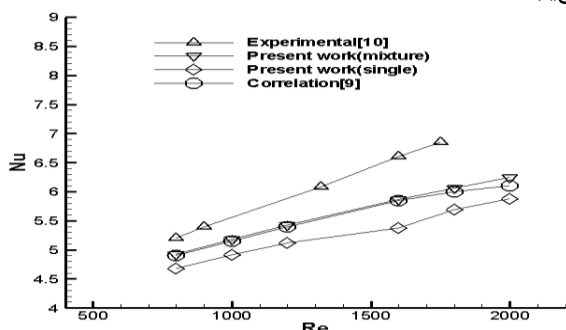
شکل ۵- تغییرات عدد ناسلت محلی در x=0.698m برحسب عدد رینولدز در کسر حجمی ۰/۰۴
