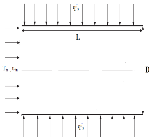
شکل ۱- هندسه مسئله و شرط مرزی
