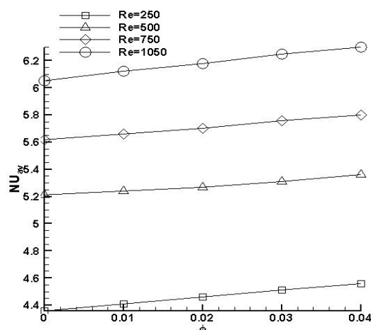
شکل ۴- تغییرات عدد ناسلت متوسط برحسب کسر حجمی در اعداد رینولدز مختلف با استفاده از مدل مخلوط در حالت شار ثابت
