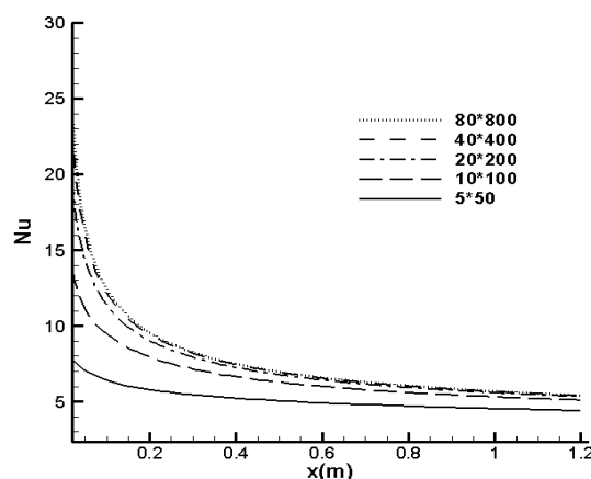
شکل ۲- بررسی استقلال نتایج از شبکه در رینولدز ۲۰۰۰ و کسر حجمی ۰/۰۴
