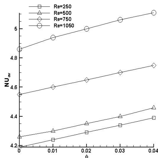
شکل ۶- تغییرات عدد ناسلت متوسط بر حسب کسر حجمی در اعداد رینولدز مختلف با استفاده از مدل مخلوط در حالت دما ثابت
