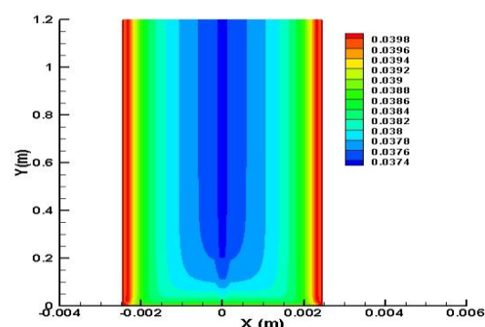
شکل ۳- توزیع کسر حجمی در رینولدز ۱۰۵۰ و کسر حجمی ۰/۰۴
