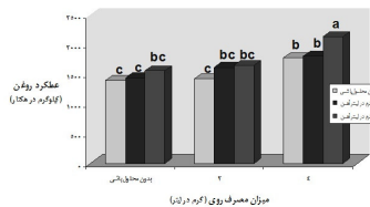
شکل ۳- برهمکنش محلول‌پاشی روی و آهن برای عملکرد
