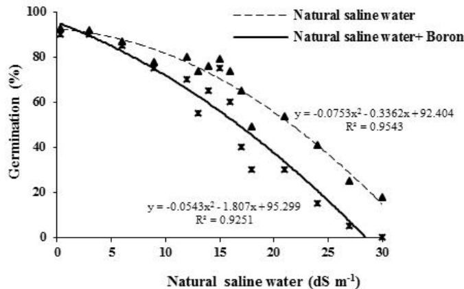
شکل ۳. تاثیر آب شور طبیعی یا تنهایی یا همراه بور بر جوانه زنی بذر کلزا
