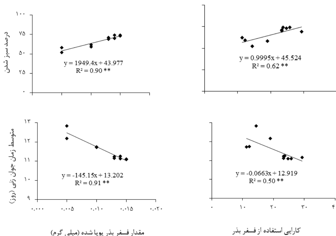
شکل ۱- ارتباط بین مقدار فسفر بذر پویا شده و کارایی استفاده از فسفر بذر با درصد و متوسط زمان سبز شدن بذرهای سیاه‌دانه
